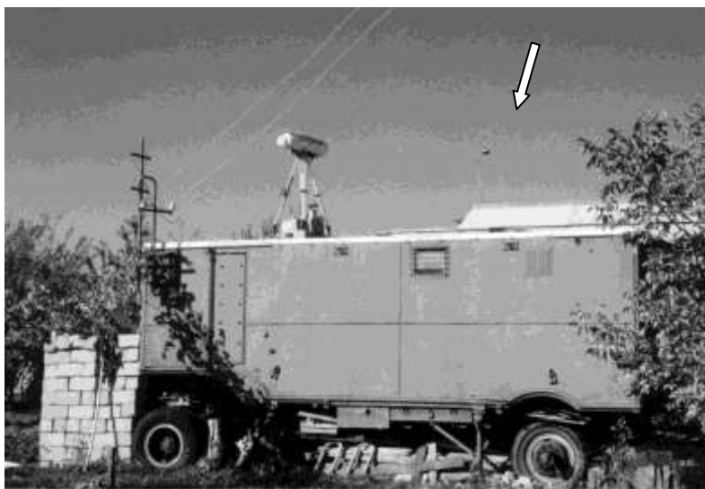
Рис.4. Оптический измерительный пункт
