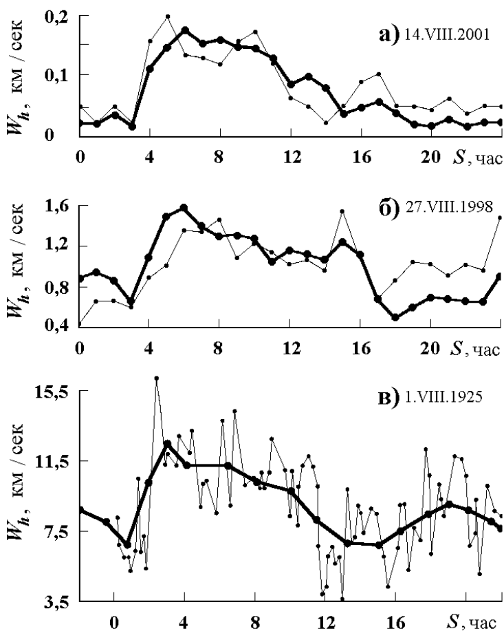
Рис.5. Изменение скорости эфирного ветра в течение суток в эпоху августа
