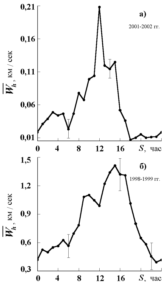
Рис.7. Средний суточный ход скорости эфирного ветра в течение звездных суток
