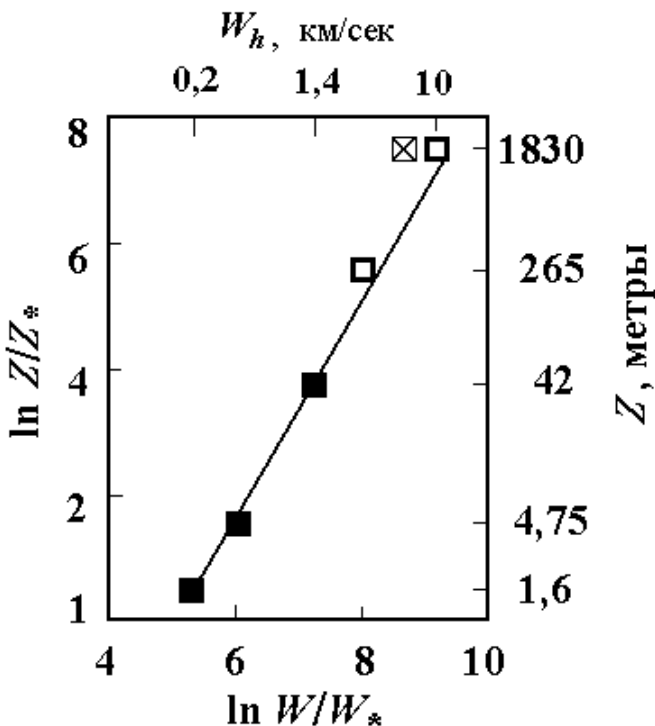
Рис.6. Зависимость скорости эфирного ветра от высоты над земной поверхностью
